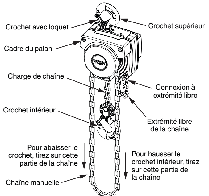
Figure 2 - Composantes principales du palan Coffing® LHH-NC
